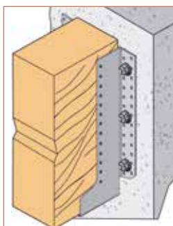
GLI : Fixation sur support BÉTON
